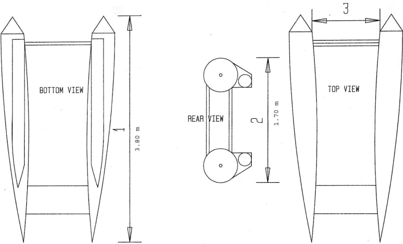
HULL DIAGRAM A:
